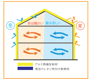
発砲ウレタン遮熱工法
