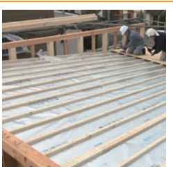
2重屋根工法
